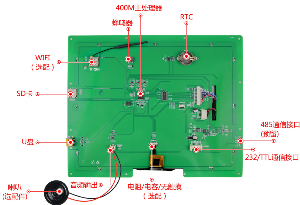
图 1-4 硬件配置图
