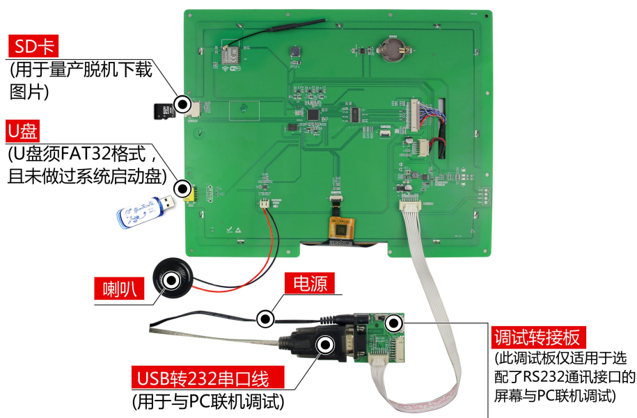
图 1-5 调试工具图
