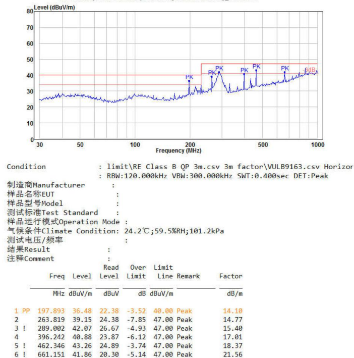
图 5-6 辐射测试水平方向
