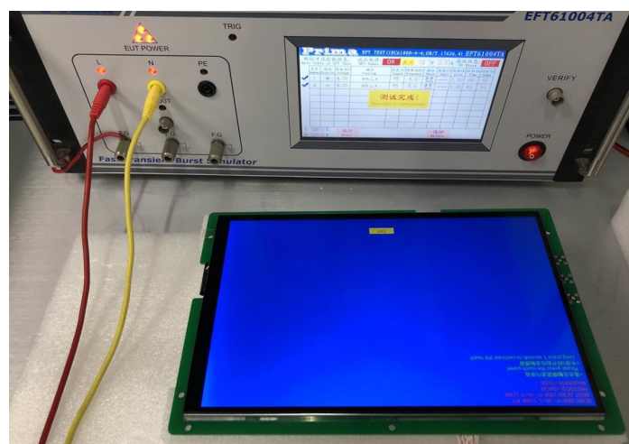
图 5-4 群脉冲测试图
